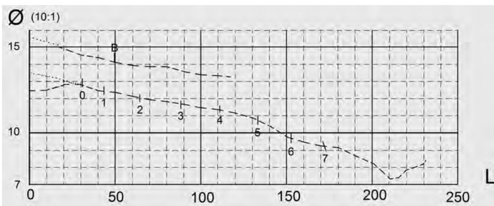
ABBILDUNG 9 Bohrungsgrafik der Sopranblockflöte von Terton. Die obere punktierte Linie der Kopfbohrung (B=Blocklinie) zeigt den vermuteten Bohrvorgang im Bereich der Schnabelkurve. Die untere Linie kennzeichnet das Bohrungsprofil vom Unterteil des zweiteiligen Instruments. Die Zahlen 0 bis 7 bezeichnen die Fingerlochpositionen; Loch 7 ist etwas schief nach unten gebohrt. Zwischen L 0 und L 25 ist die Zapfenkontraktion gut zu sehen. Der rekonstruierte Verlauf der Bohrung ist punktiert abgebildet. Im Kopf verjüngt sich die Bohrung von 14,1 mm bei der Blocklinie bis auf 13,1 mm am unteren Ende am Zapfenherz (welches nicht in der Grafik eingezeichnet ist). Im Unterteil erweitert sich die Bohrung im Bereich der Zapfenkontraktion von 12,5 auf 12,9 mm, um dann schmaler zu werden. Nach Loch 5 ist die Verjüngung stärker, während sich die Bohrung auf den letzten 20 mm wieder erweitert. An der schmalsten Stelle beträgt der Bohrungsdurchmesser 7,2 mm.
