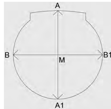
ABBILDUNG 11 Querschnitt durch den Blockflötenkopf im Kernspaltbereich A–A 1 : der vertikale Bohrungsdurchmesser (Ø-ver) B–B 1 : der horizontale Bohrungsdurchmesser (Ø-hor)
