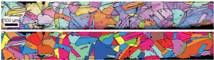
ABILDUNG 11 Resultate der EBSD-Untersuchung vom Schall von Instrument Nr. 2. Oben Überlagerung von inverser Polfigur und REM-Bild. Mitte individuelle Färbung der Körner mit Korngrenzen, darunter Korngrößenverteilung und Statistik
