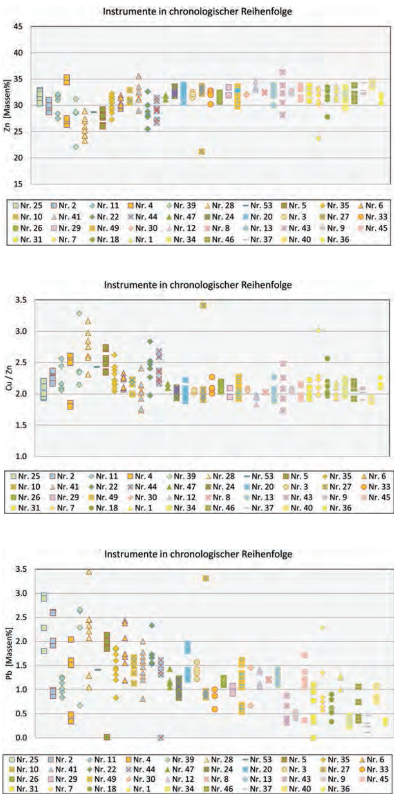
ABBILDUNG 3-5 Entwicklung des Zinkgehalts (oben), des Kupfer-Zink-Verhältnisses (Mitte) und des Bleigehalts (unten) in französischen Blechblasinstrumenten im 19. Jahrhundert. Die Nummern beziehen sich auf die Instrumentenliste, gleiche Farben markieren gleiche Hersteller.
