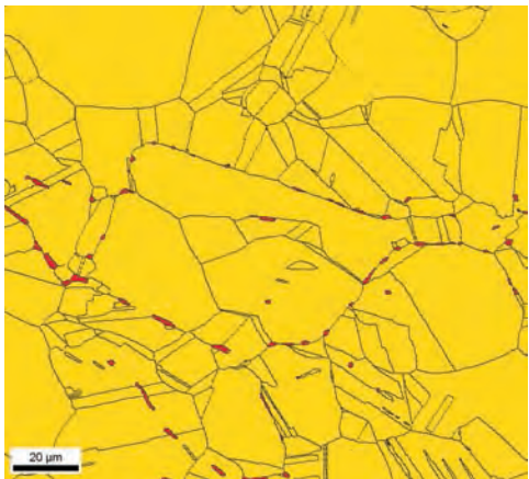
ABILDUNG 13 EBSD-Untersuchung. Unten Bild mit Korngrenzen und Phasenbestand, rechts Legende. In Gelb \alpha -Messing, in Rot das zinkreichere \beta -Messing
